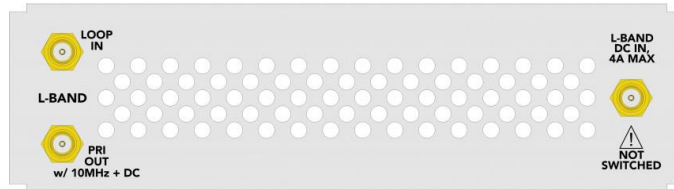
Рисунок 8. Модуль SMD 940
